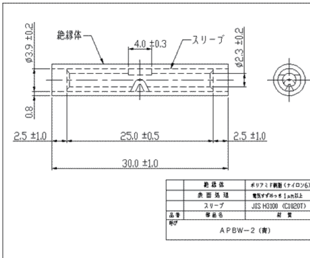
APBW-2 (青) 図面
