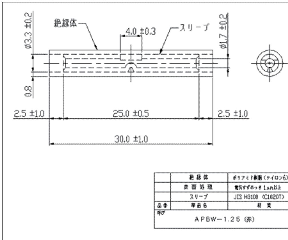
APBW-1.25 (赤) 図面
